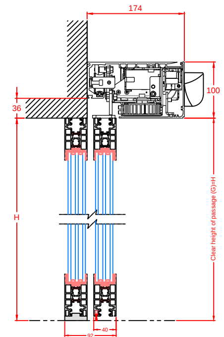
Section A-A
