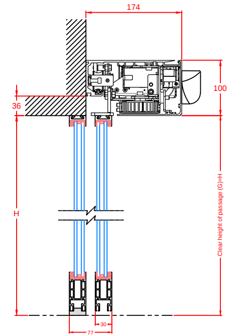
Section A-A
